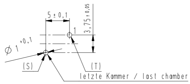
Lochbild für 250V / hole pattern for 250V = B
