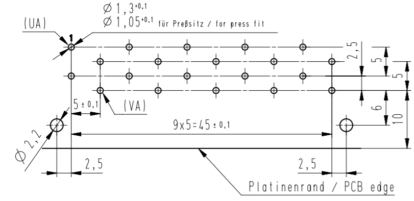
Lochbild (Bestückungsseite) / hole pattern (component side)
