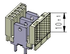
Farbkennzeichnungsbereich bei versilberten Kontakten colour coding area when silvered contacts (nach / according WN 30.70 Bereich / area "D")
