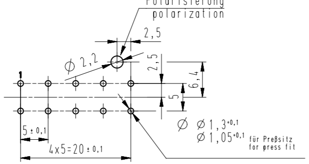
Lochbild (Bestückungsseite) / hole pattern (component side)
