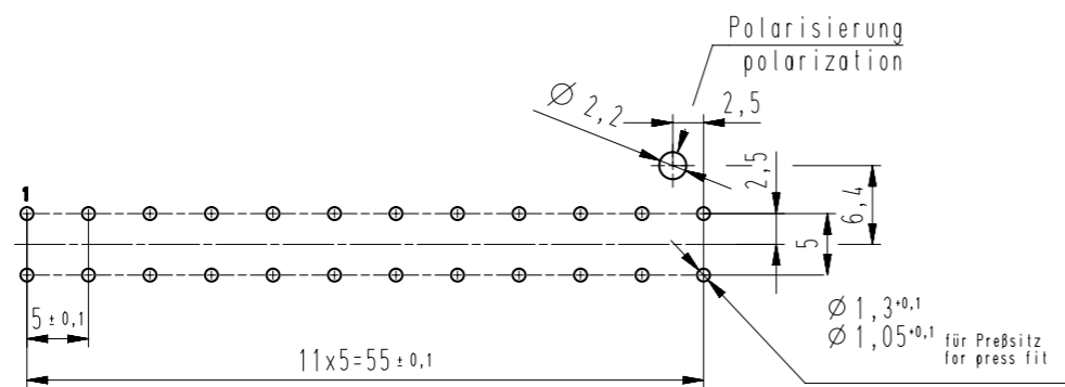
Lochbild (Bestückungsseite) / hole pattern (component side)
