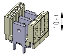
Farbkennzeichnungsbereich bei versilberten Kontakten colour coding area when silvered contacts (nach / according WN 30.70 Bereich / area "D")
