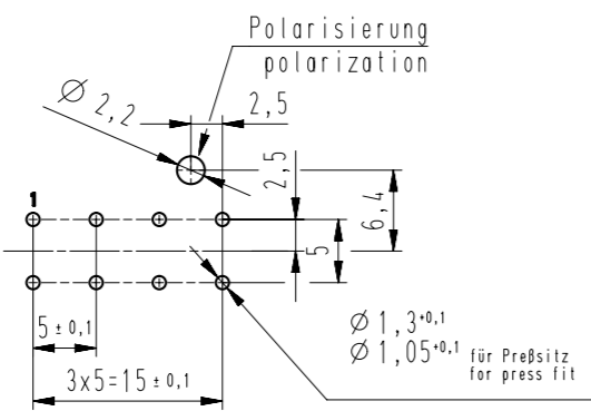
Lochbild (Bestückungsseite) / hole pattern (component side)
