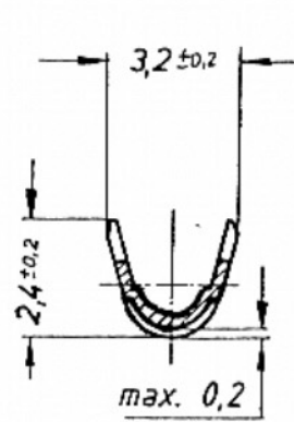
Schnitt C-D
