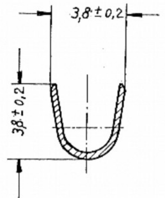
Schnitt A-B
