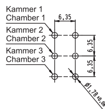
Lochbild von der Bestückungsseite Hole pattern viewed from component side
