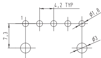
Beispiel Leiterplatte 5-polig / Sample PCB 5 poles
