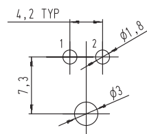
Leiterplatte 2-polig / PCB 2 poles
